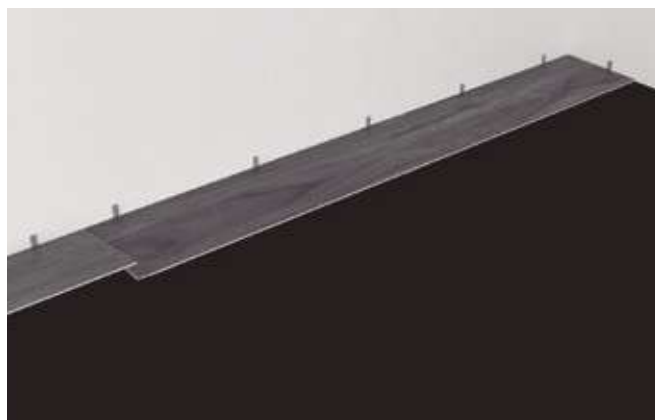
Paso 1: Primer tablón, primera fila. Coloque un espaciador de 3/8" (9,525mm) de grosor a la izquierda y coloque la tabla contra la pared.
