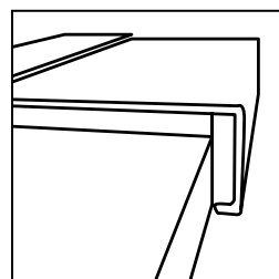
SQUARE FLUSH STAIR NOSE NARIZ DE ESCALERA CUADRADA A RAS
