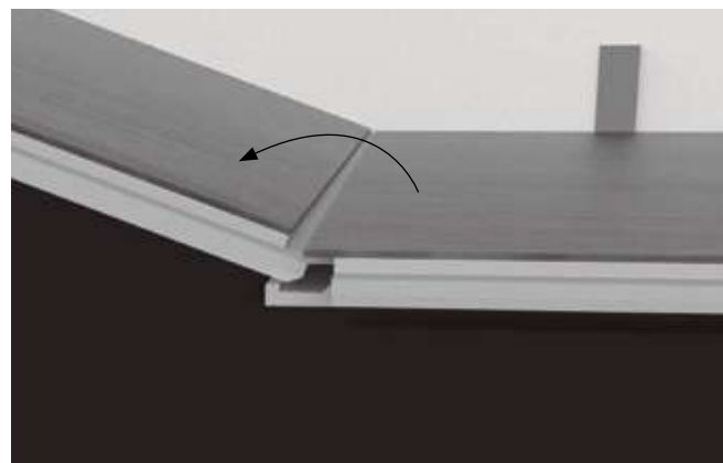
Paso 2: Segunda tabla, primera fila. Coloque esta tabla suavemente y apretada en el extremo corto de la primera.
