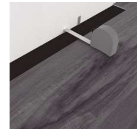
Paso 10: Última fila. El ancho mínimo de la última tabla no debe ser MENOR de 2" de ancho. Coloque un separador antes de medir. Corte los paneles a lo largo y pegue los extremos cortos..
