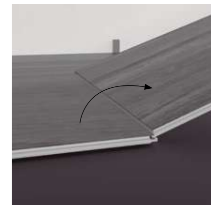
Paso 8a: Segunda tabla, segunda fila. Coloque el panel en ángulo en la ranura de la fila anterior asegurándose de que el extremo del panel esté apretado / alineado con el extremo corto del panel anterior.
