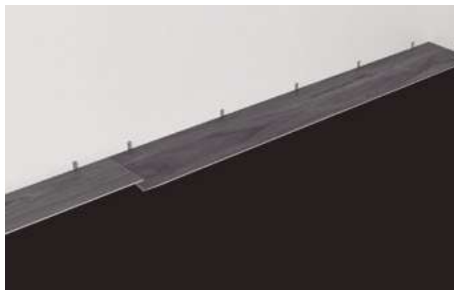
Paso 3: Doble el panel hacia abajo en un solo movimiento de acción. Luego presione hacia abajo o toque ligeramente hacia abajo en el extremo corto que acaba de instalar hasta que haga clic..
