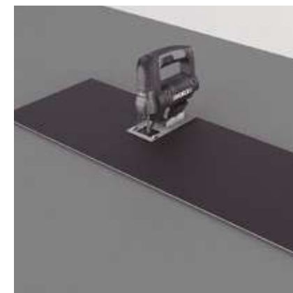
Paso 5: Corte con una sierra de calar, sierra de mano, sierra de corte o cortador de guillotina. Luego, rompa el piso, de manera similar a los paneles de yeso.
