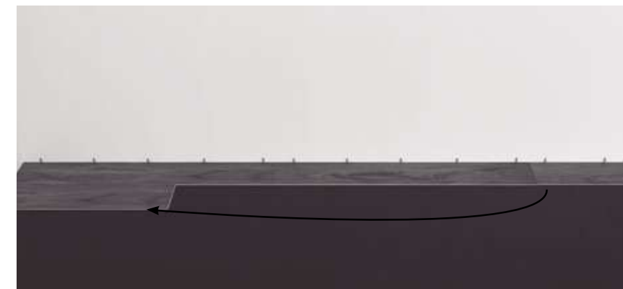
Paso 6: Comenzando la segunda fila, la primera tabla debe tener una longitud mínima de 10" (254 mm). Coloque un espaciador de 3/8" (9,525 mm) contra la pared y mida la última pieza. Si es más corto que 10" (254 mm), se debe usar una nueva pieza de arranque. Inserte en ángulo en la fila anterior y tóquelo (en el lado largo) con un bloque de golpeo hasta que quede plano.
