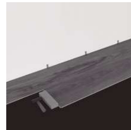
Paso 8c: El producto está correctamente bloqueado cuando las dos tablas están al ras en la parte superior. Termine de instalar este tablón golpeándolo con un bloque de golpeo en el lado largo para garantizar una instalación segura.
