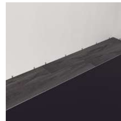
Paso 7: La distancia mínima entre los extremos cortos de las tablas en filas paralelas no debe ser inferior a 6" (152,4 mm).
