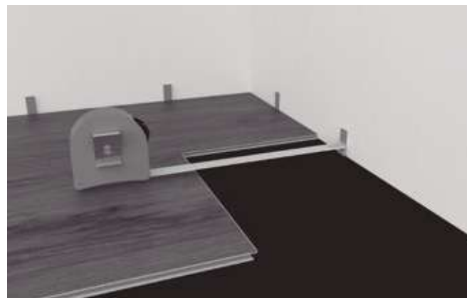
Paso 4: Al final de la primera fila, coloque un espaciador de 3/8" (9,525 mm) en la pared y mida la longitud del último tablón para que encaje.
